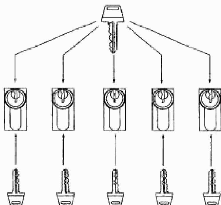
Рисунок Б.3 — Система цилиндровых механизмов с групповым ключом — группа механизмов, каждый из которых можно открывать и закрывать как собственным ключом, так и групповым ключом, свойственным для данной группы
