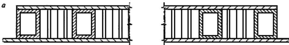
Полотно с двумя стальными листами, стальными профилями коробчатого сечения и сотовым наполнением
