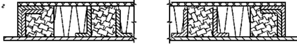
Полотно с наружным стальным листом и внутренним листом из ДВП, уголковыми стальными профилями с брусками из древесины и заполнением из пенопласта
