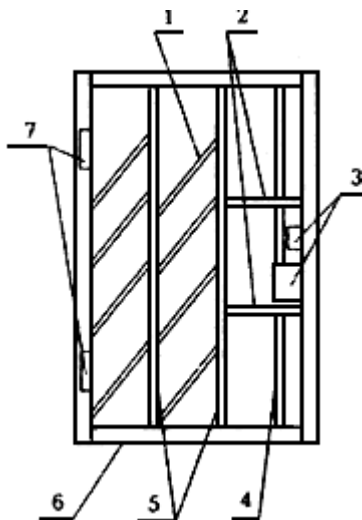
1 - наклонные усиливающие профили; 2 - горизонтальные усиливающие профили; 3 - запирающие элементы; 4 - металлический короб для тяг; 5 - вертикальные усиливающие профили; 6 - профиль обвязки полотна; 7 - петли
