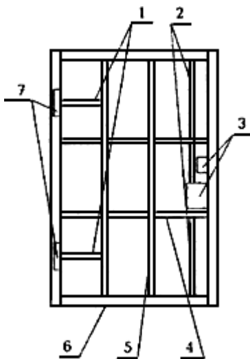
1 - горизонтальный усиливающий профиль под петли; 2 - металлический короб для тяг; 3 - запирающие элементы; 4 - горизонтальный усиливающий профиль; 5 - вертикальный усиливающий профиль; 6 - профиль обвязки полотна; 7 - петли
