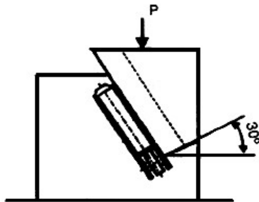
Рисунок В.1 - Схема приложения статической нагрузки на верхнюю петлю
