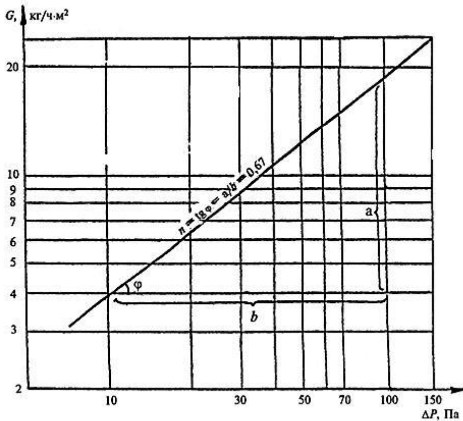
Рисунок 3 - Пример построения диаграммы зависимости массовой воздухопроницаемости от перепада давления
