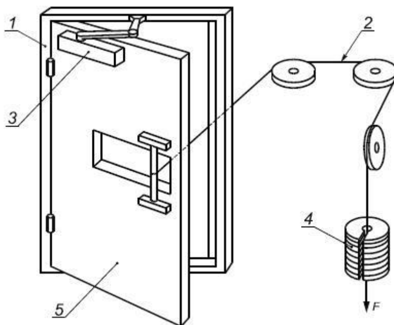
Рисунок Д.1 - Пример устройства для проведения испытаний доводчиков на безотказность
