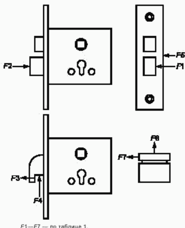
Рисунок 1 — Точки приложения сил, воздействующих на механизм замка
